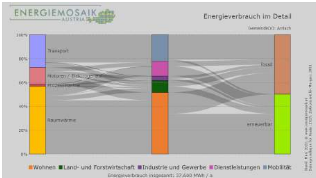
Abbildung 15 Primärenergieverbrauch Arriach 23
